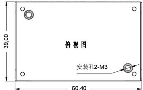
标准型 60.4*39.0*12.7mm
